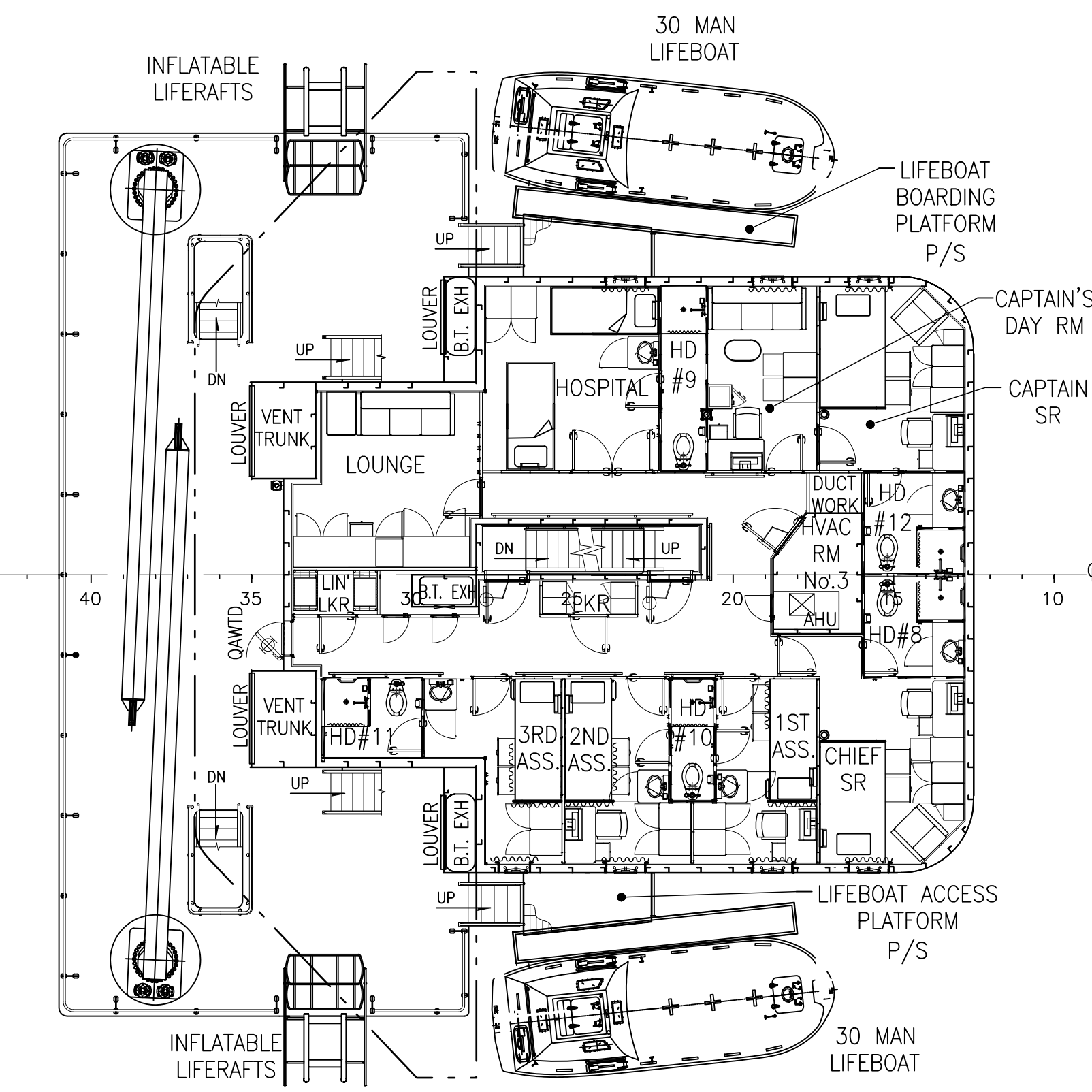
02 DECK SCALE: 1/8"=1'-0"
