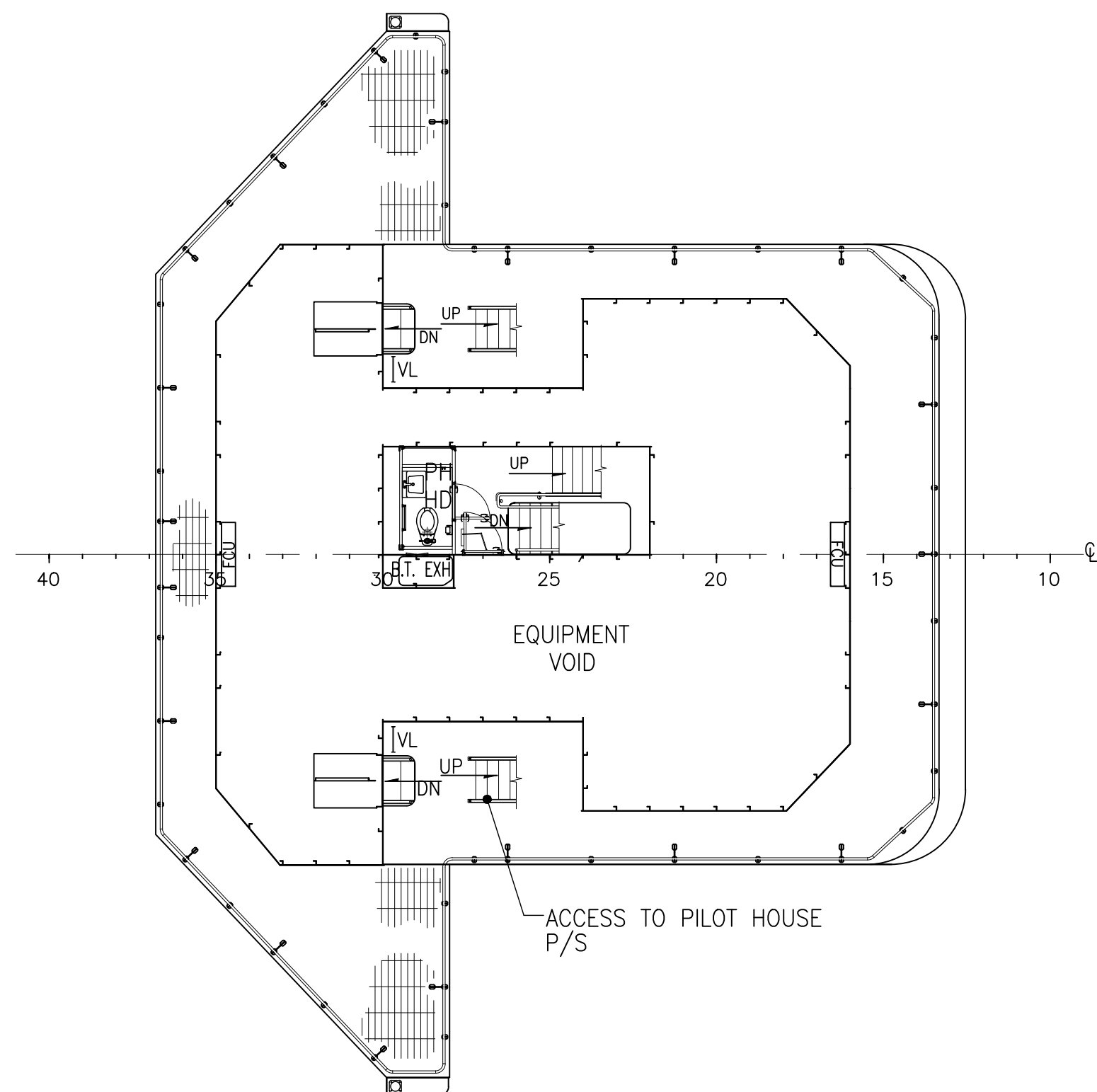
03 DECK SCALE: 1/8"=1'-0"
